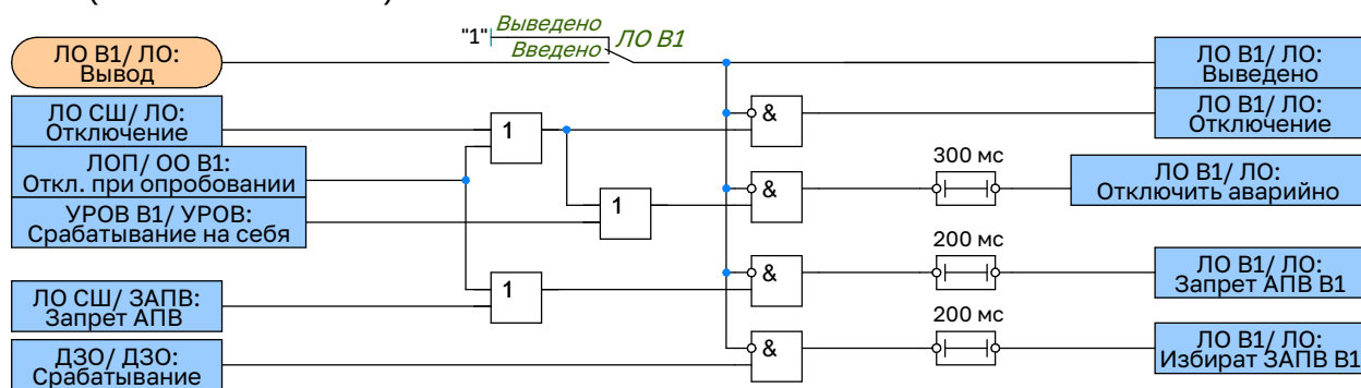
Рисунок 2.13 – Функциональная схема логики отключения В1
